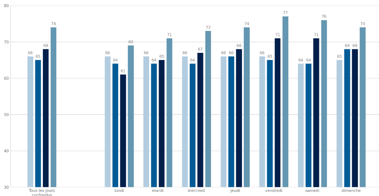
Paris 13 - Quai d'Austerlitz - Point 3 Variation quotidienne du niveau sonore en dB(C) Saison 2023
