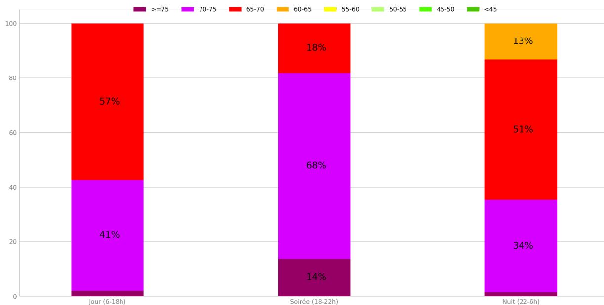
Paris 13 - Port de la Gare - Point 5 Distribution des niveaux sonores moyens en dB(C) par plage Saison 2023
