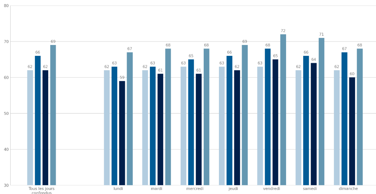
Paris 13 - Port de la Gare - Point 5 Variation quotidienne du niveau sonore en dB(C) Saison 2023
