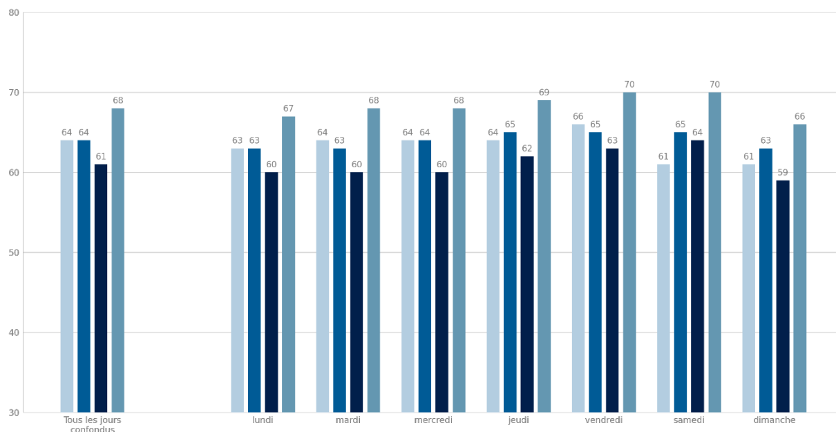
Paris 13 - Port de la Gare - Point 1 Variation quotidienne du niveau sonore en dB(C) Saison 2023
