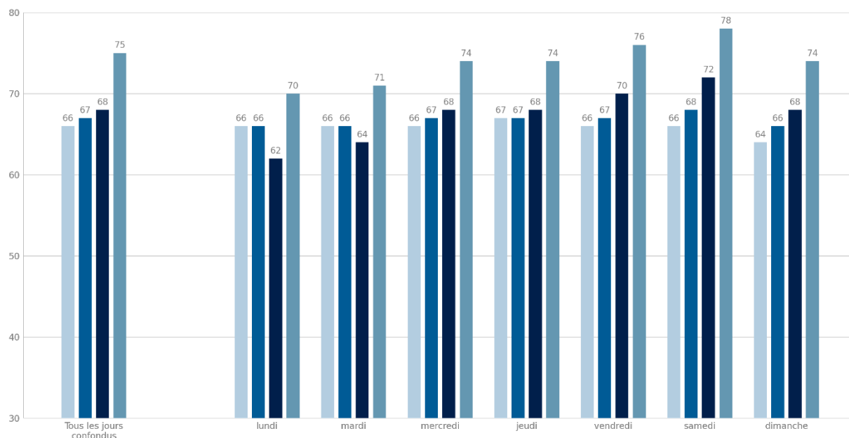
Paris 12 - Port de la Rapée - Point 4 Variation quotidienne du niveau sonore en dB(C) Saison 2023
