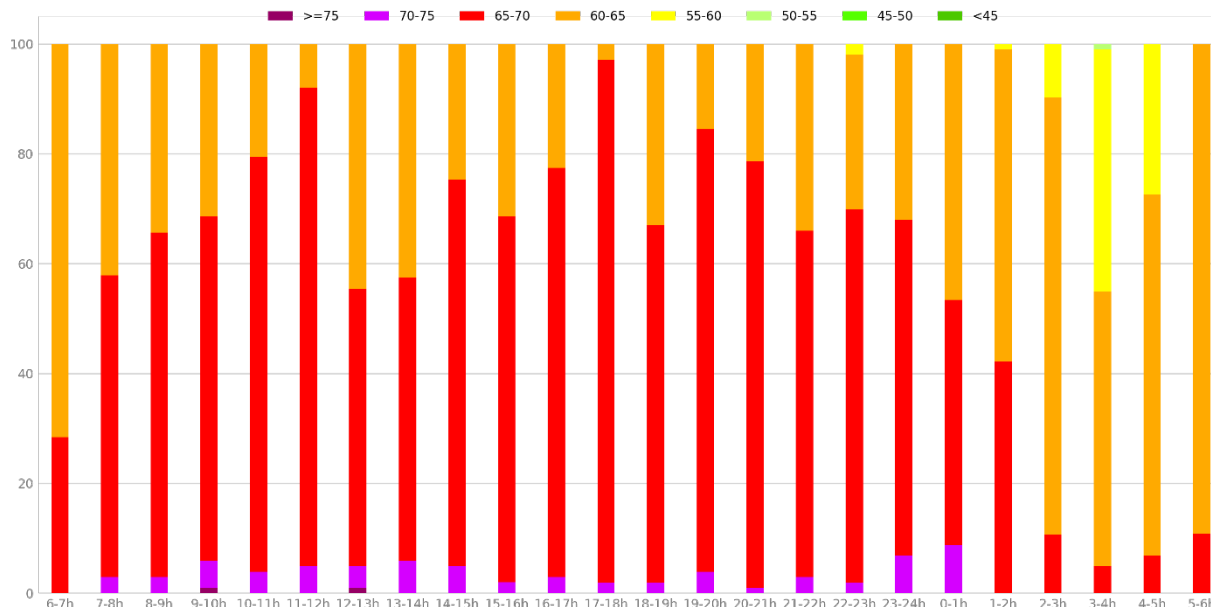
Paris 12 - Port de Bercy - Point 1 Distribution des niveaux sonores moyens en dB(C) par plage Saison 2023
