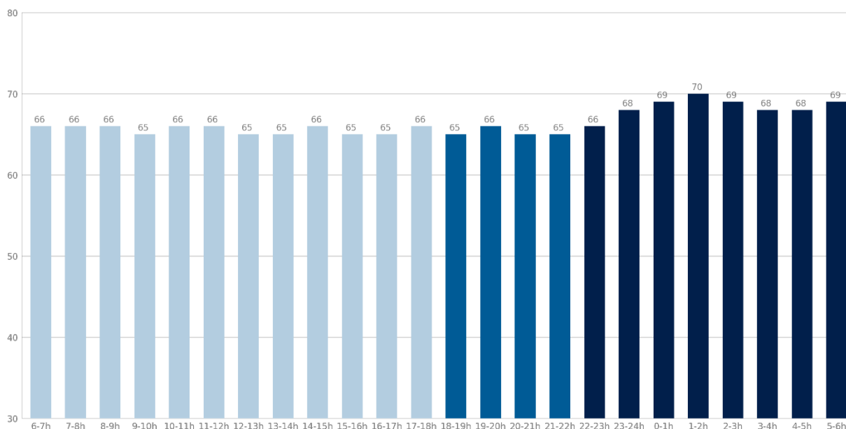
Paris 13 - Quai d'Austerlitz - Point 3 Niveaux sonores moyens en dB(C) par plage Saison 2023
