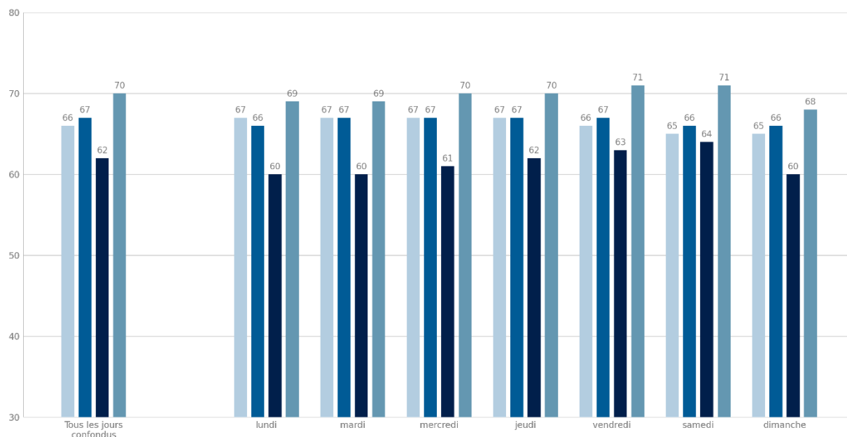
Paris 13 - Quai d'Austerlitz - Point 1 Variation quotidienne du niveau sonore en dB(C) Saison 2023
