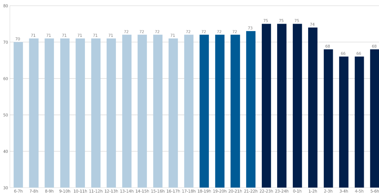
Paris 12 - Port de la Rapée - Point 4 Niveaux sonores moyens en dB(C) par plage Saison 2023
