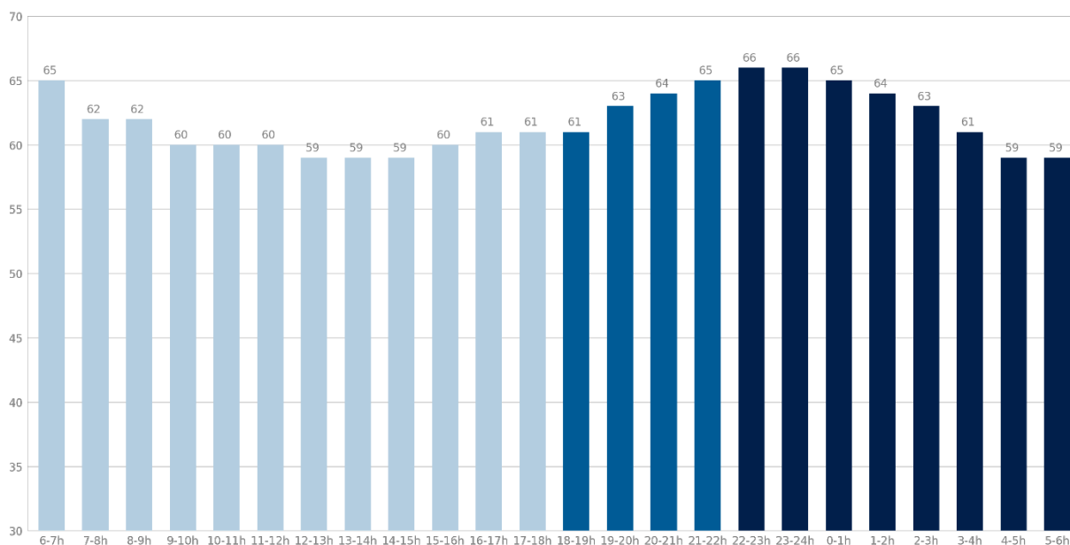
Paris 13 - Port de la Gare - Point 6 Niveaux sonores moyens en dB(C) par plage Saison 2023
