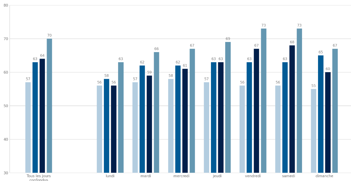
Paris 13 - Quai d'Austerlitz - Point 2 Variation quotidienne du niveau sonore en dB(C) Saison 2023
