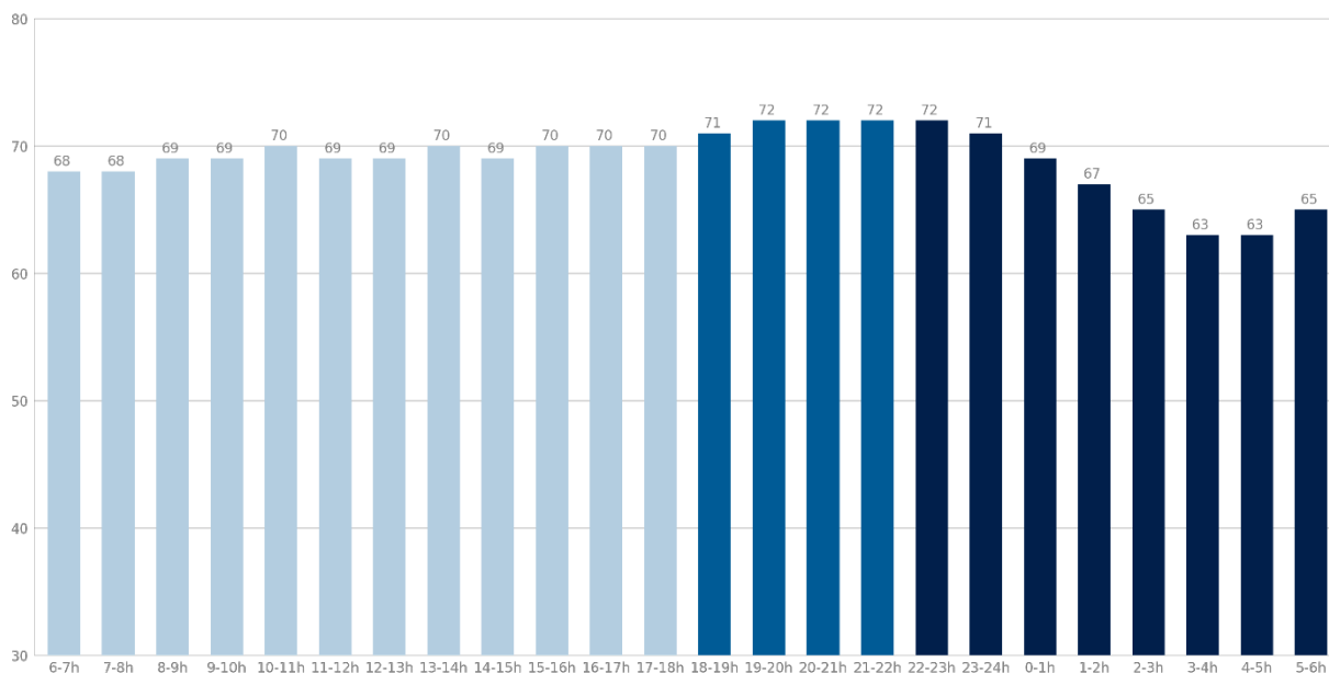
Paris 13 - Port de la Gare - Point 7 Niveaux sonores moyens en dB(C) par plage Saison 2023
