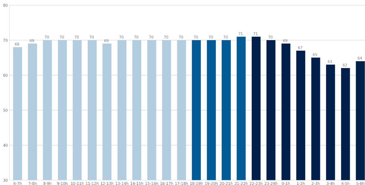
Paris 13 - Port de la Gare - Point 1 Niveaux sonores moyens en dB(C) par plage Saison 2023
