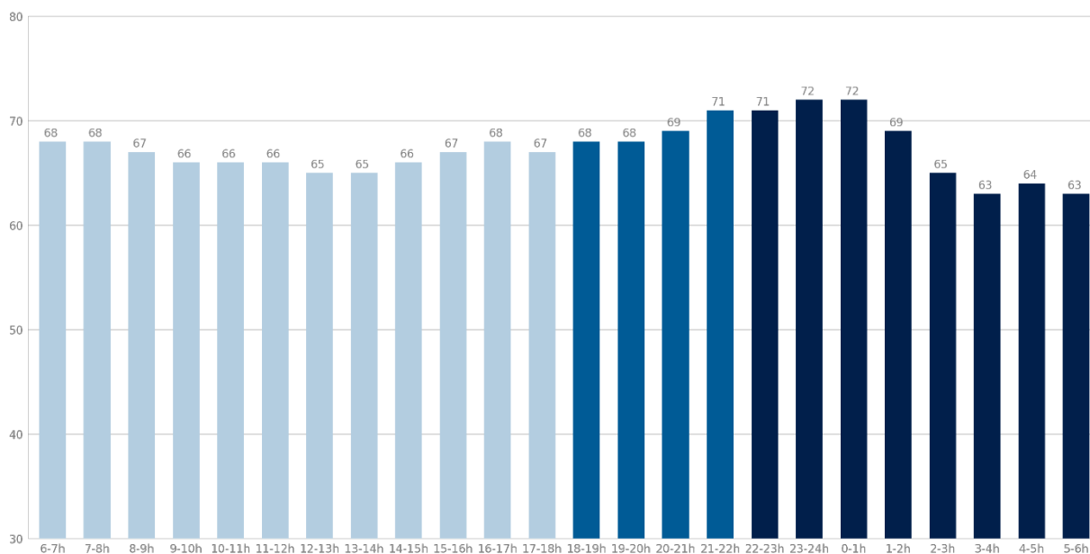
Paris 12 - Port de la Rapée - Point 1 Niveaux sonores moyens en dB(C) par plage Saison 2023
