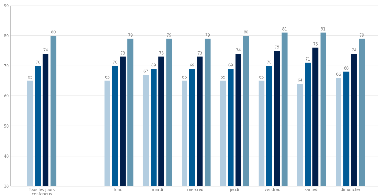
Paris 12 - Port de la Rapée - Point 2 Variation quotidienne du niveau sonore en dB(C) Saison 2023
