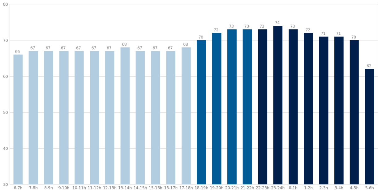
Paris 13 - Quai d'Austerlitz - Point 2 Niveaux sonores moyens en dB(C) par plage Saison 2023
