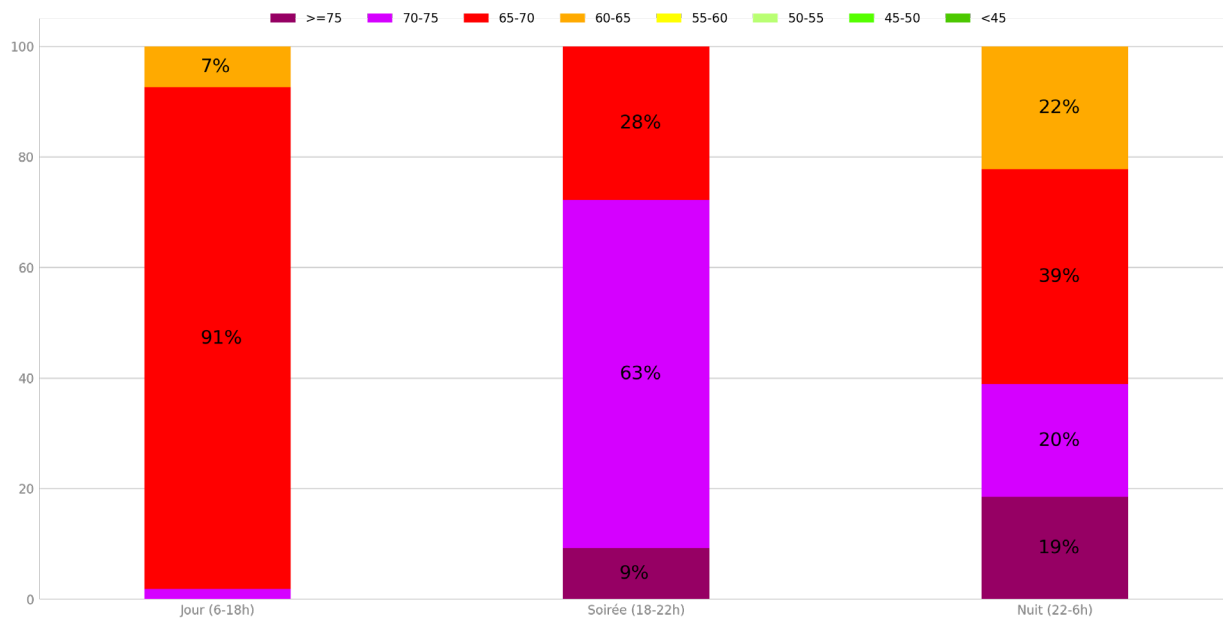
Paris 13 - Quai d'Austerlitz - Point 2 Distribution des niveaux sonores moyens en dB(C) par plage Saison 2023
