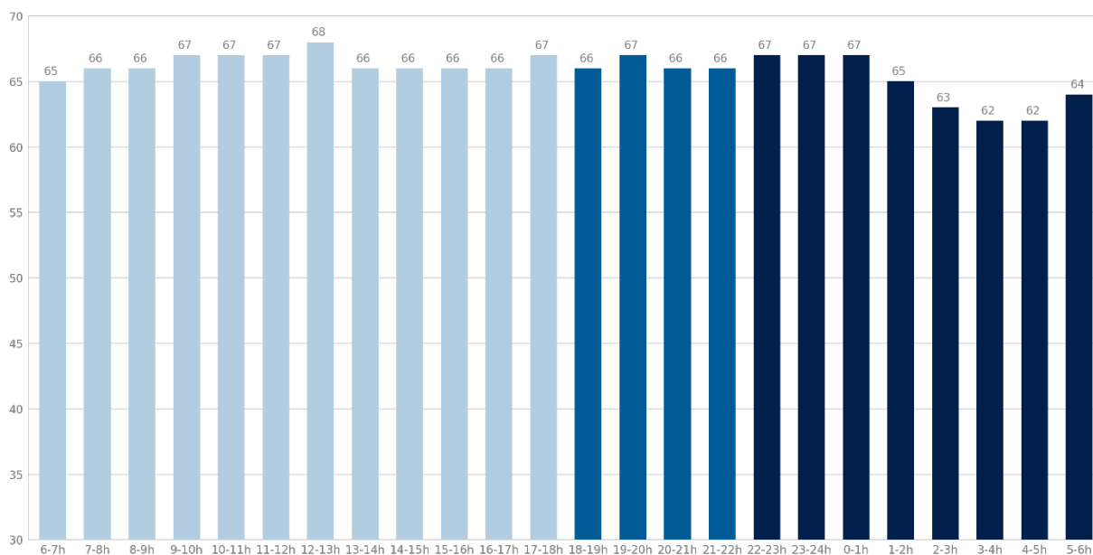
Paris 12 - Port de Bercy - Point 1 Niveaux sonores moyens en dB(C) par plage Saison 2023
