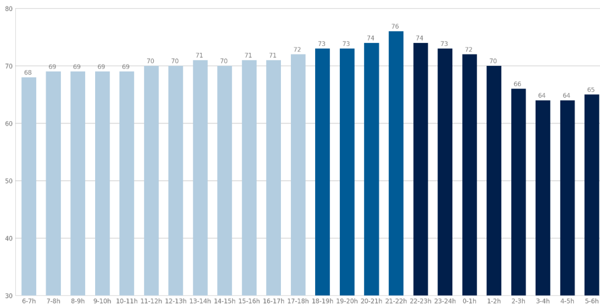
Paris 13 - Port de la Gare - Point 5 Niveaux sonores moyens en dB(C) par plage Saison 2023
