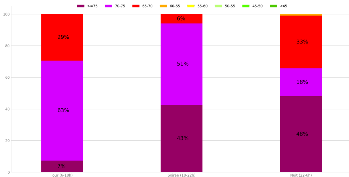
Paris 12 - Port de la Rapée - Point 2 Distribution des niveaux sonores moyens en dB(C) par plage Saison 2023
