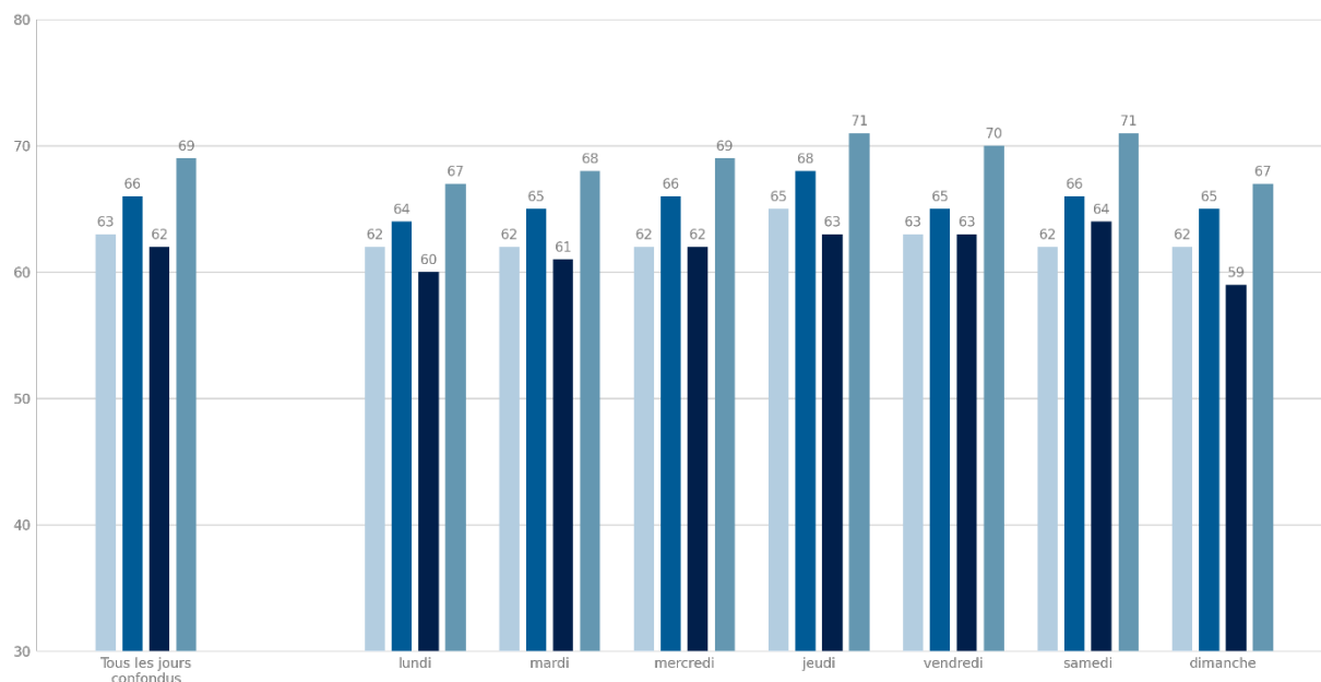
Paris 13 - Port de la Gare - Point 7 Variation quotidienne du niveau sonore en dB(C) Saison 2023
