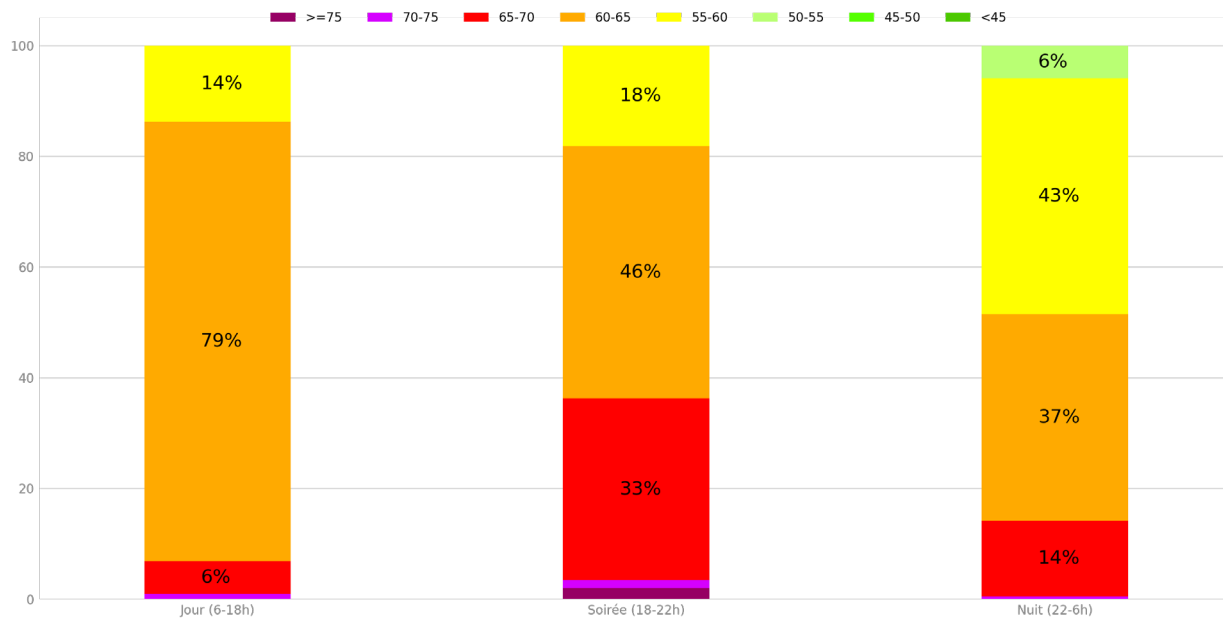
Paris 13 - Port de la Gare - Point 5 Distribution des niveaux sonores moyens en dB(A) par plage Saison 2023
