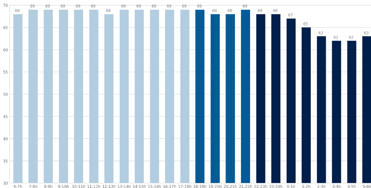
Paris 13 - Port de la Gare - Point 3 Niveaux sonores moyens en dB(C) par plage Saison 2023
