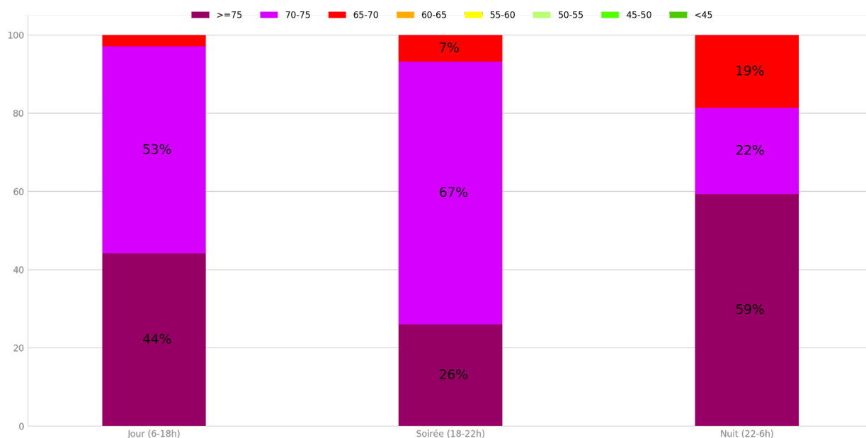
Paris 13 - Quai d'Austerlitz - Point 3 Distribution des niveaux sonores moyens en dB(C) par plage Saison 2023
