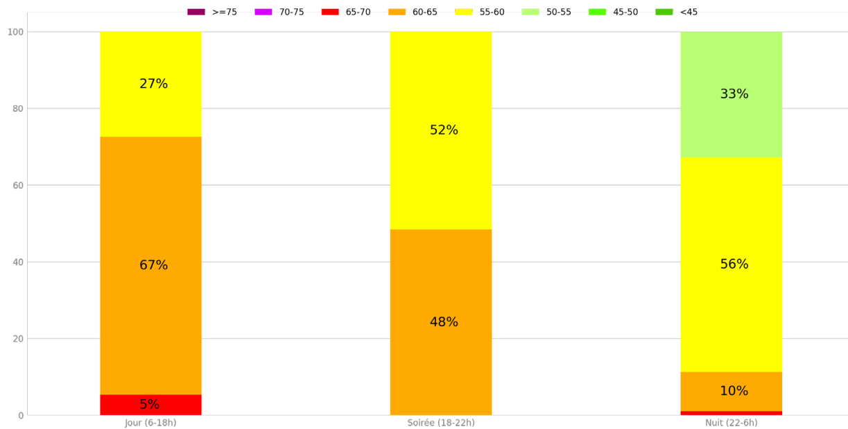
Paris 13 - Port de la Gare - Point 3 Distribution des niveaux sonores moyens en dB(A) par plage Saison 2023
