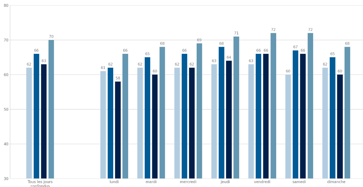
Paris 13 - Port de la Gare - Point 4 Variation quotidienne du niveau sonore en dB(C) Saison 2023
