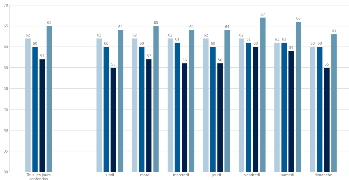
Paris 13 - Port de la Gare - Point 3 Variation quotidienne du niveau sonore en dB(C) Saison 2023
